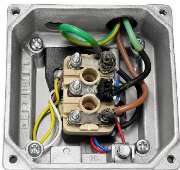
Conexión defectuosa
