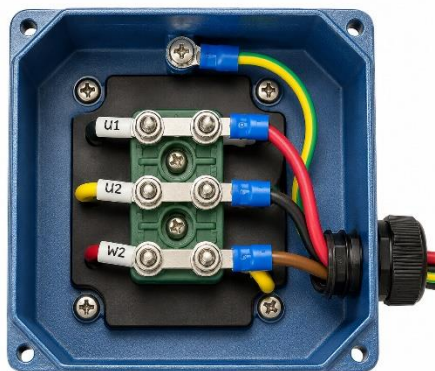
Conexión correcta
