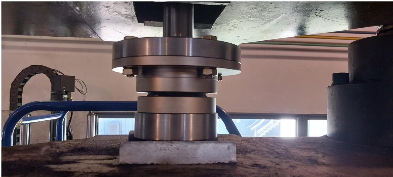
Figura 1: Metodología utilizada para el ensayo solicitado
